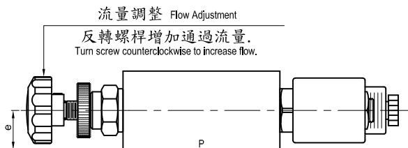
尺寸 Dimensions(mm)
